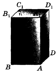
Прямоугольный параллелепипед
