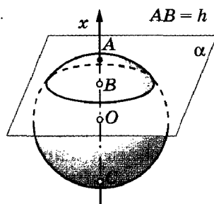
Шаровой сегмент
