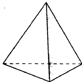
Правильный тетраэдр
