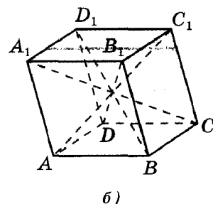
Параллелепипед
