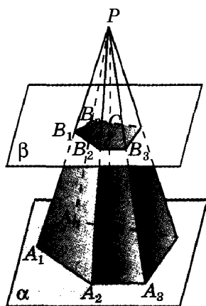
Усеченная пирамида
