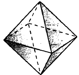
Октаэдр
