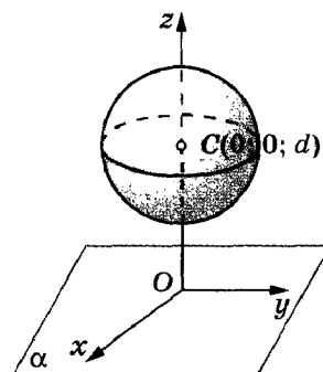
d > R в)
