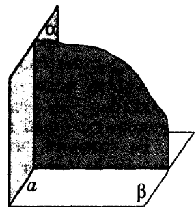
Если \gamma \perp a , то \gamma \perp \alpha и \gamma \perp \beta
