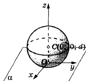
d = R б)
