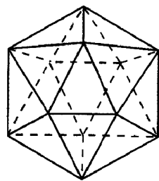
Правильный икосаэдр
