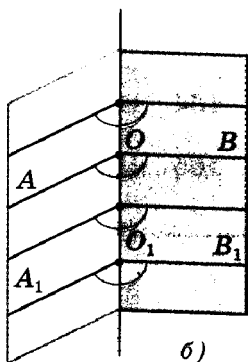
Линейный угол двугранного угла
