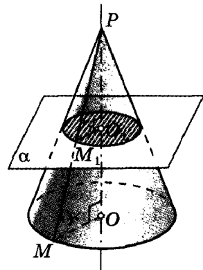
Сечение конуса плоскостью \alpha , перпендикулярной к его оси, — круг с центром O_1 радиуса r_1 = \frac{PO_1}{PO}r Рис. 152
