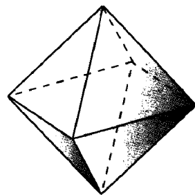
Правильный октаэдр
