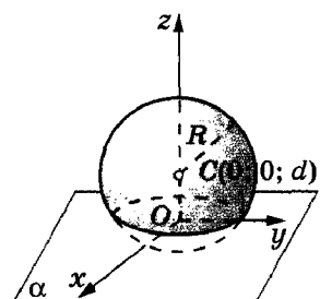
d < R, r = \sqrt{R^2 - d^2} а)
