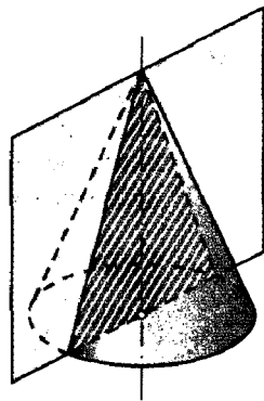
Осевое сечение конуса Рис. 151
