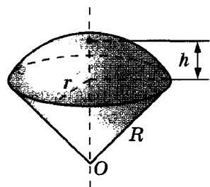
Шаровой сектор
