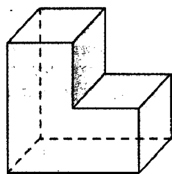
Невыпуклый многогранник
